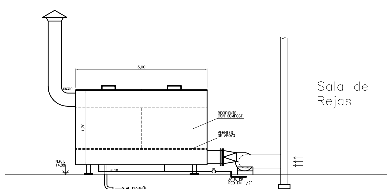
CORTE AA
