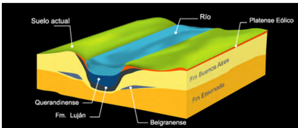
Figura 11: Esquema de formaciones pospampeana y pampeana
