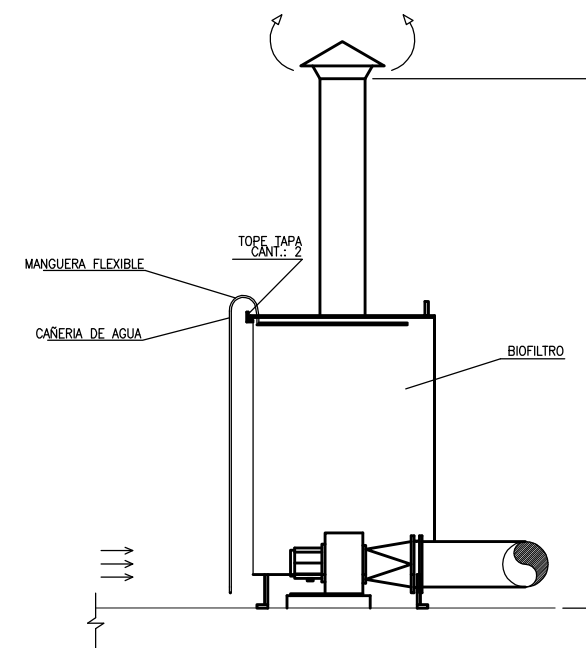
CORTE BB
