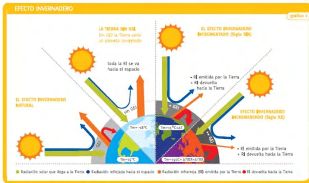
Figura 24: Diferentes escenarios posibles del efecto invernadero
