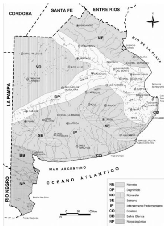
Figura 12: Regiones hidrogeológicas de la Provincia de Buenos Aires
