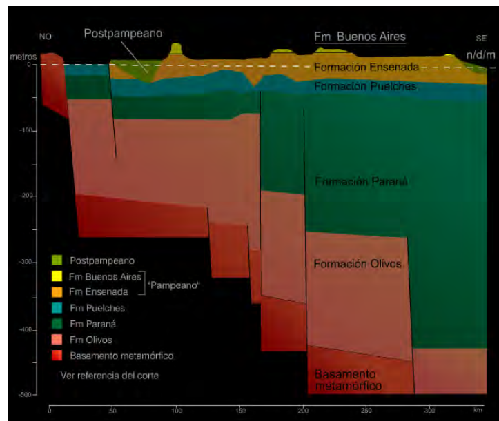
Figura 10: Esquema de corte estratigráfico suelo – subsuelo
